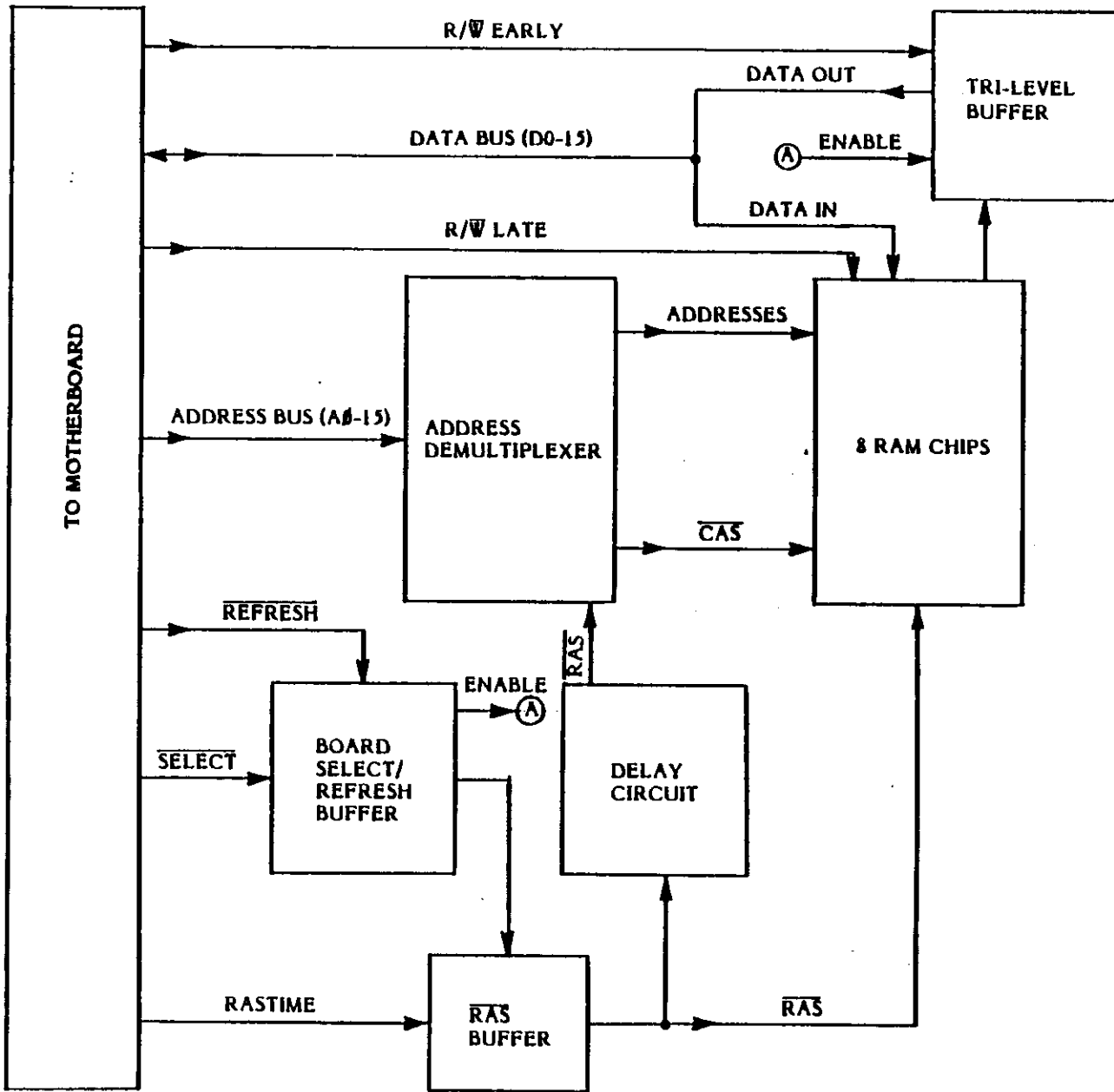
16K DYNAMIC RAM ATARI
